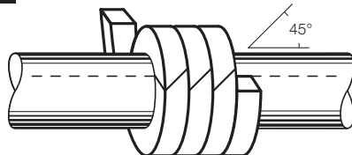
図1 バイアスカット（リング2本の構成）
